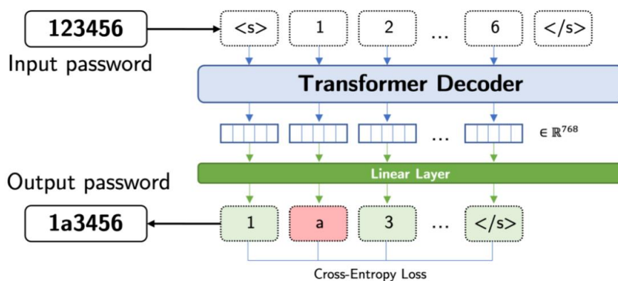
Рис.5. Прогнозування моделлю PassGPT вхідного символу в позиції n з використанням попередніх токенів. Зелений колір вказує на правильне прогнозування; червоний – на неправильне [13].
