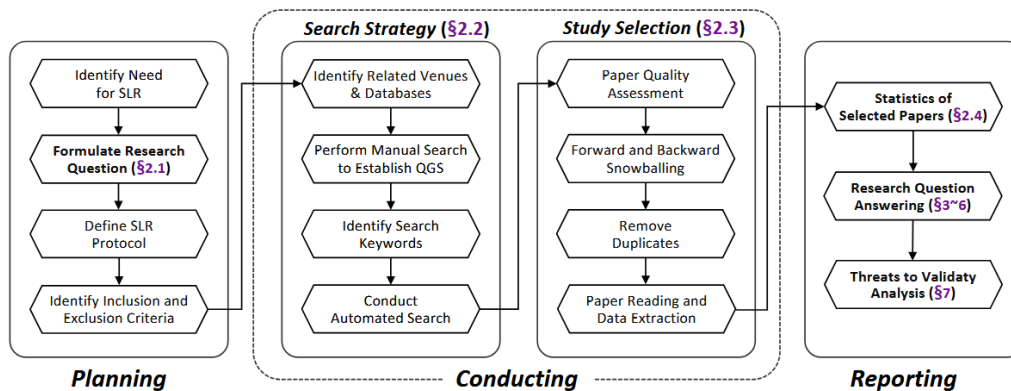
Рис.9. Схема систематичного огляду літератури для LLM4Security [17].
